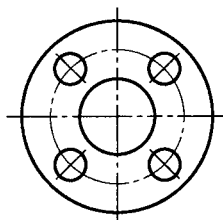
图 8 法兰螺栓孔的跨中布置
