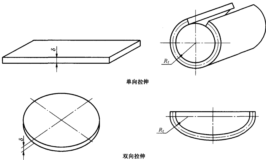
图 12 单向拉伸和双向拉伸成形
