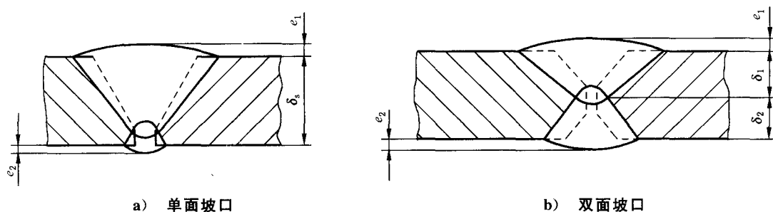
图 11 A、B 类焊接接头的焊缝余高
