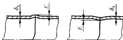
图6 焊接接头处的轴向棱角
